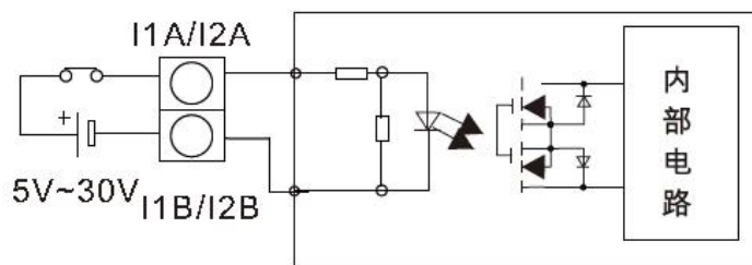
图 6. 触发输入电路连接示意图
