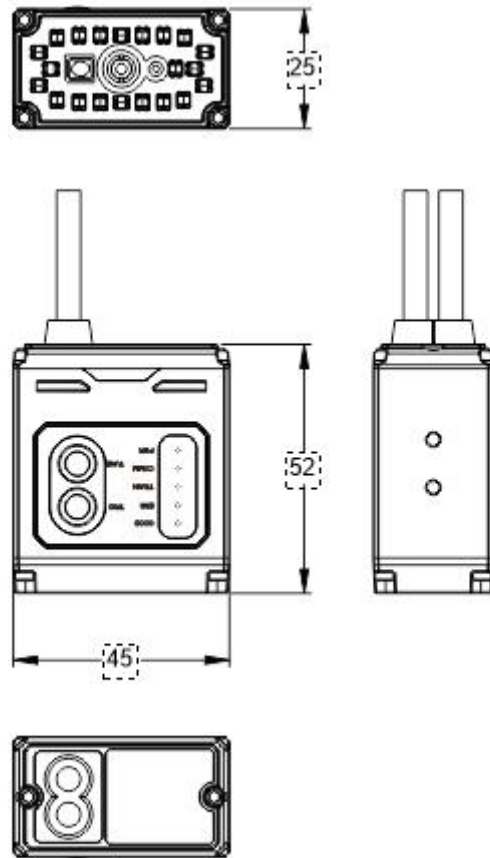
图 2. Soldier100 外观尺寸图
