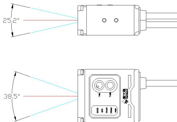
图 5. Soldier100 识读角度示意图
