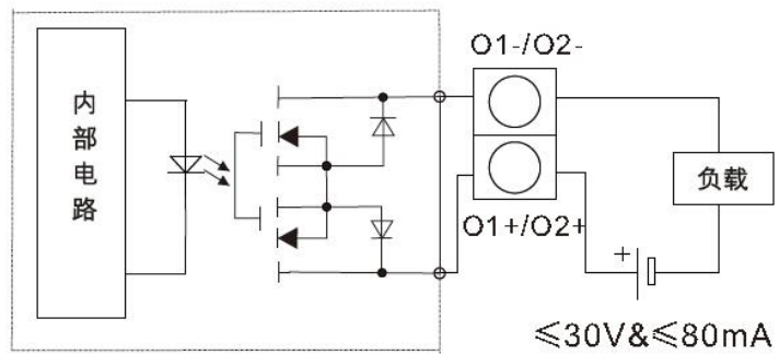
图 7. 指示信号输出电路连接示意图
